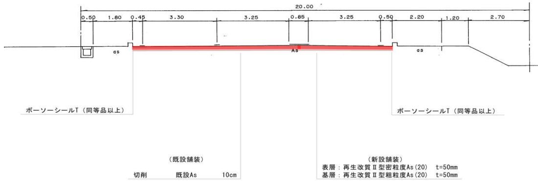
標準断面図
